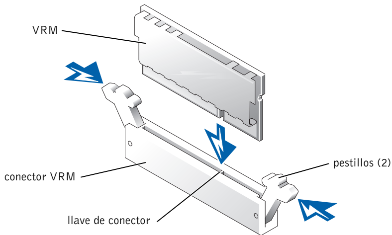
Figura 7-2. Instalación del VRM
