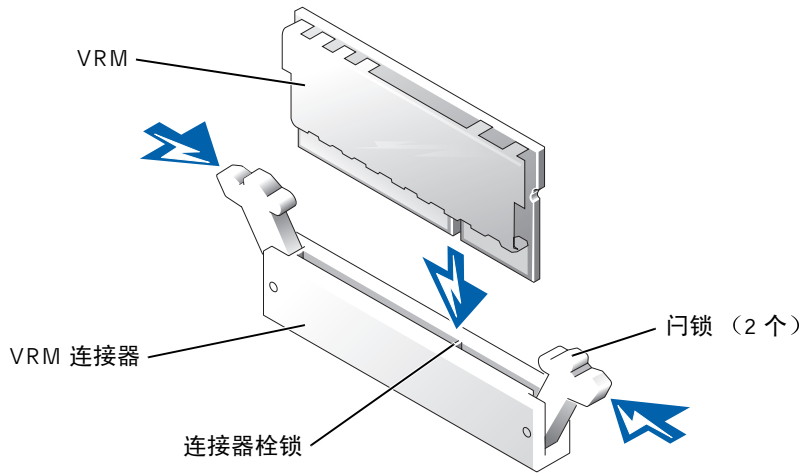
图 2-2：安装 VRM
