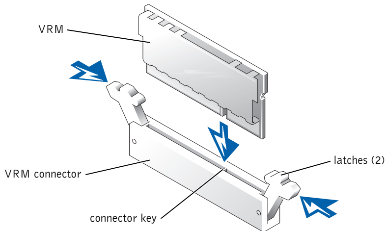
Figure 3-2. Installation d'un module VRM
