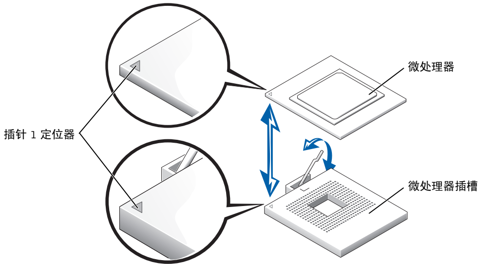
图 2-1：卸下和更换微处理器
