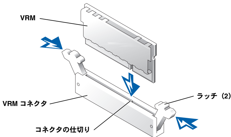
図 5-2. VRM の取り付け
