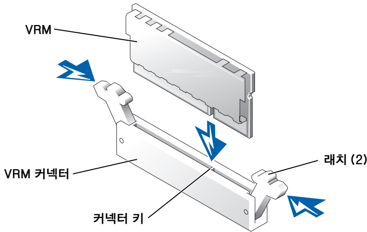
그림 6-2. VRM 설치
