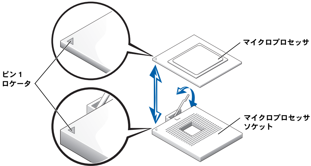
図 5-1. マイクロプロセッサの取り外しと交換
